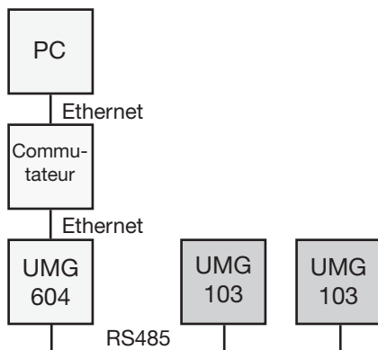
Fig. Raccordement de plusieurs UMG103 à un PC par un UMG604 (avec l'option Ethernet).
