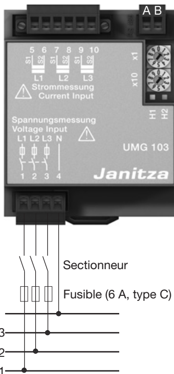
Fig. Exemple de raccordement : Mesure de la tension par des sectionneurs et des fusibles.
