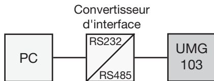
Fig. Raccordement d'un UMG103 par un PC par le biais d'un transformateur d'interface.
