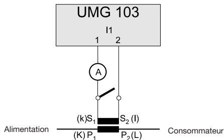
Fig.: Exemple de mesure d'intensité par un ampèremètre supplémentaire.
