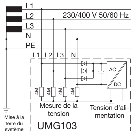
Fig. Schéma de principe, UMG103 dans le réseau TN.
