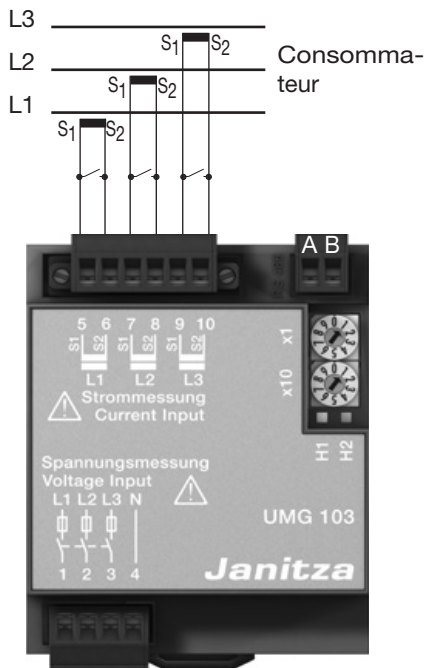
Fig.: Exemple de raccordement, mesure d'intensité par transformateur d'intensité.
