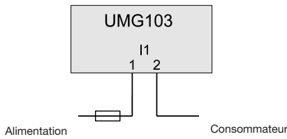
Fig.: Exemple, mesure directe de la tension
