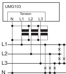
Fig. Exemple de raccordement pour la mesure de la tension par des transformateurs de tension.
