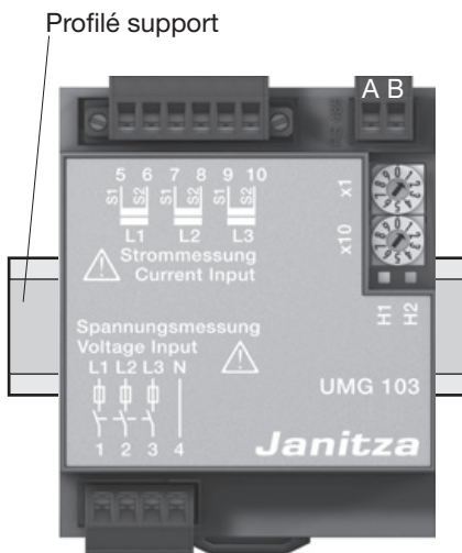
Fig. UMG103 sur support profilé selon DIN EN 60715.
