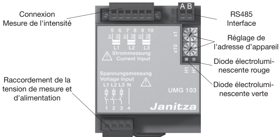
Fig.: Vue de l'UMG103.
