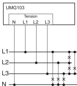
Fig. Exemple de raccordement pour une mesure directe de la tension.
