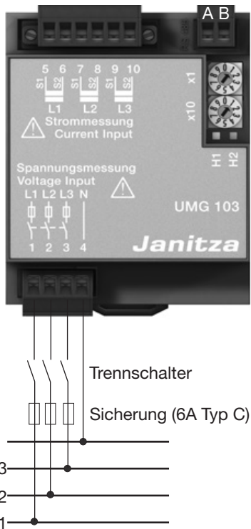
Abb. Anschlussbeispiel: Spannungsmessung über Trennschalter und Sicherungen.
