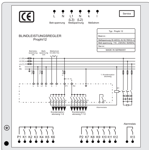
Bild 2: Prophi12 Rückansicht
