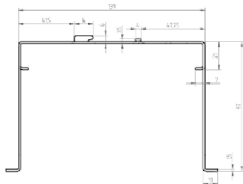
Vorderansicht
