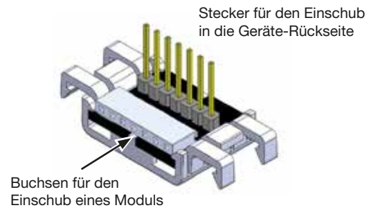
Busverbinder
