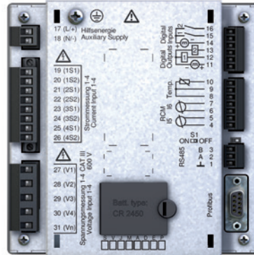
Rückansicht
