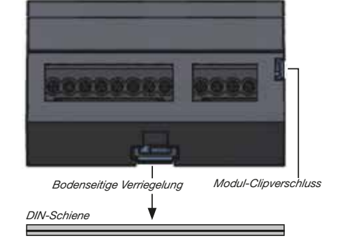
Abb. Gerät auf DIN-Schiene.
