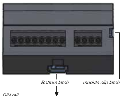
Fig. Device on DIN rail.
