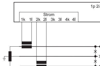
Abb. Strommessung im Einphasen-3-Leiter-system. Anschlussvariante 0 (Siehe Seite 50).
