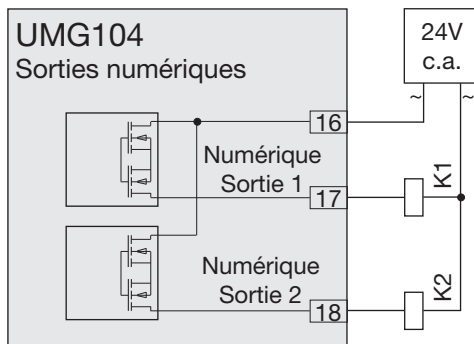
Fig. 39.1 Raccordement de relais à courant alternatif aux sorties numériques.
