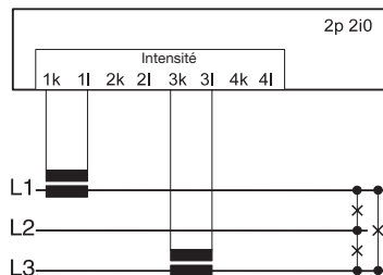
Fig. Mesure de l'intensité, exemple de raccordement pour la variante de raccordement 1 (voir page 50).
