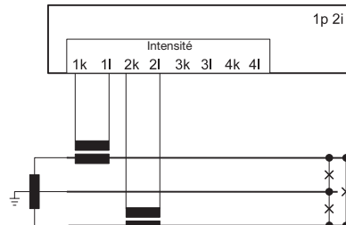
Fig. Mesure de l'intensité sur des systèmes monophasés à 3 conducteurs. Variante de raccordement 0 (voir page 50).
